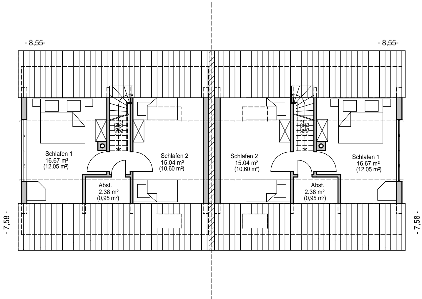
Grundriss OG, Typ 2
